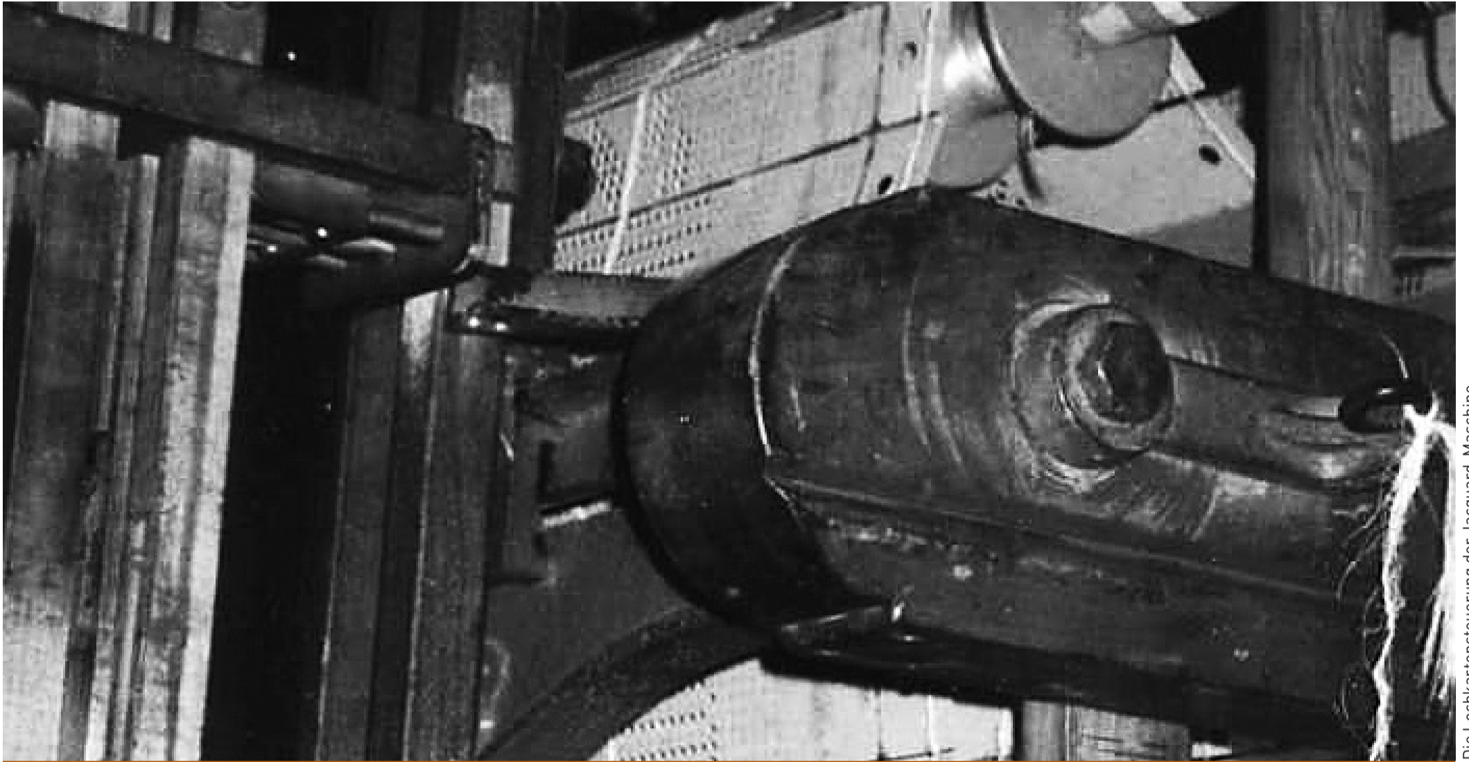
Die Lochkartensteuerung der Jacquard-Maschine
